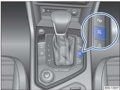
图 166 在中控台：用于手动打开全景影像系统的按钮
