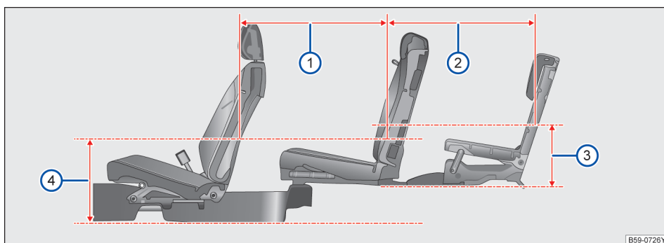
图 96 座间距
