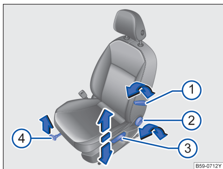
图 72 左侧前座椅上的操作元件
