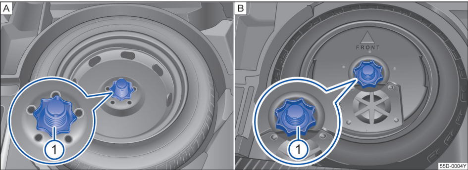
图 234 行李厢内：备用车轮固定手轮（类型 A 和类型 B）
