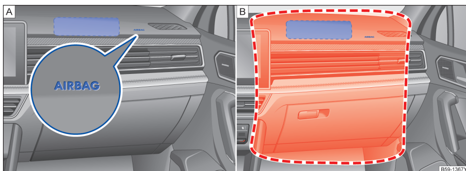
图 38 副驾驶员前部安全气囊的安装位置和膨胀范围
