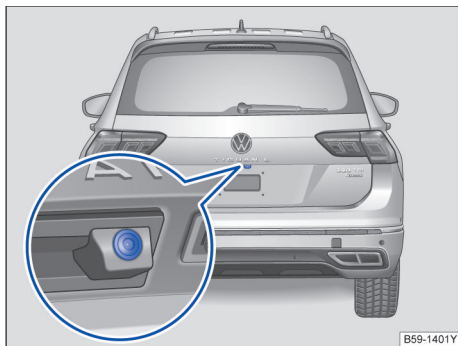
图 163 车辆行李厢盖内：倒车摄像头的安装位置
