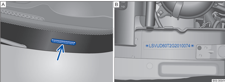
图 243 A. 车辆识别代号 B. 发动机舱内的车辆识别代号钢印位置
