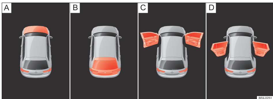
图 16 显示屏显示：[A]. 发动机舱盖处于打开状态 [B]. 行李厢盖处于打开状态 [C]. 前车门处于打开状态 [D]. 后车门处于打开状态
