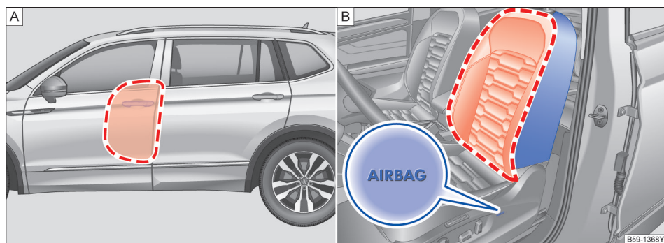
图 39 A 汽车左侧 - 侧面安全气囊膨胀范围；B 左前座椅侧面 - 侧面安全气囊安装位置及膨胀范围
