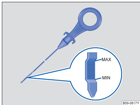
图 226 带液位标记的机油标尺
