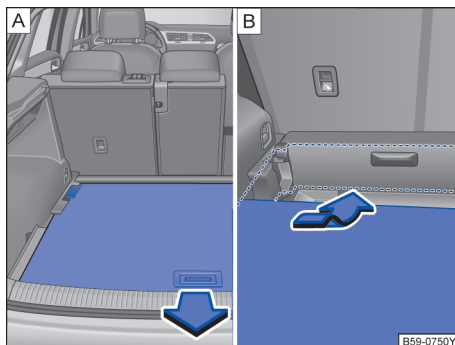
图 197 行李厢内：竖起行李厢地板（视装备而定）
