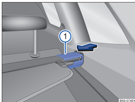
图 192 行李厢内：拆卸行李厢盖板
