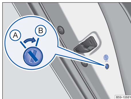
图 54 在左后车门中：儿童安全锁 A 已关闭、B 已接通
