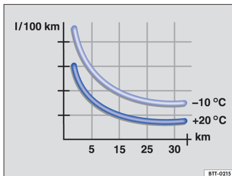
图 119 两种不同环境温度时的百公里油耗
