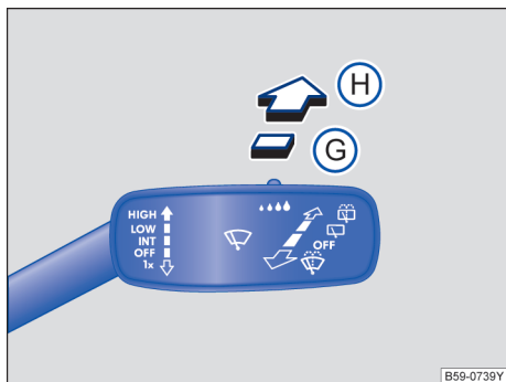
图 103 后风窗刮水器操纵杆操作位置
