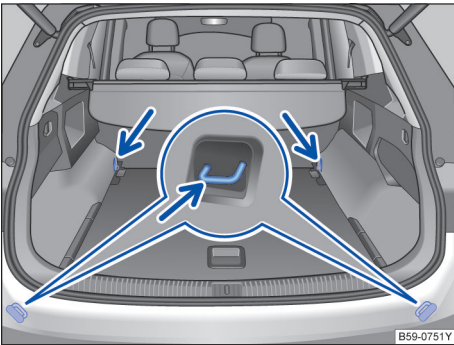
图 202 在行李厢中：固定环
