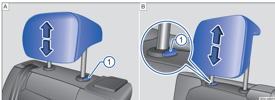
图 82 A. 调节第二排座椅头枕 B. 调节第三排座椅头枕
