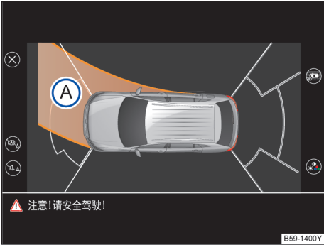
图 162 泊车雷达系统显示屏：施加转向时汽车行驶路径显示模式
