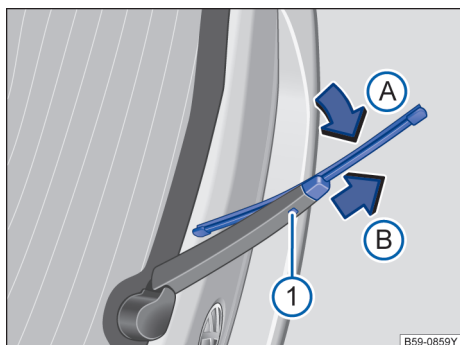
图 213 更换后风窗刮水器刮水片
