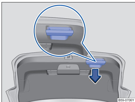
图 61 已打开的行李厢盖：用于拉动关闭的拉手
