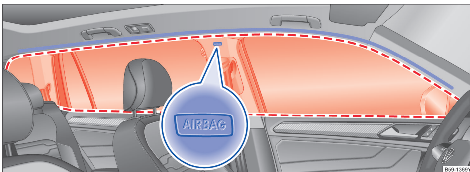
图 40 在汽车左侧：头部安全气囊的安装位置和膨胀范围
