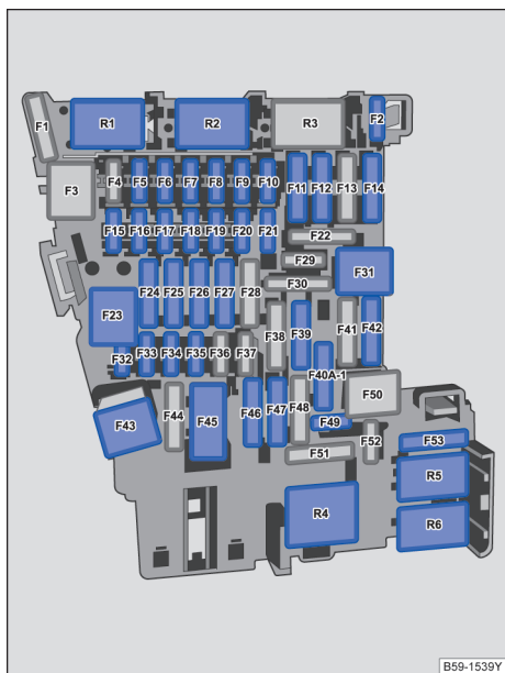
图 215 仪表板中：保险丝分配
