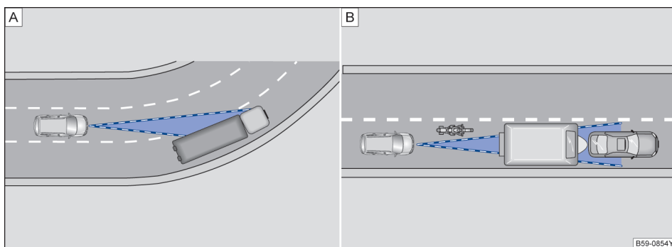
图 141 [A]. 处在弯道里的汽车 [B]. 前方行驶的摩托车处在雷达传感器探测范围外
