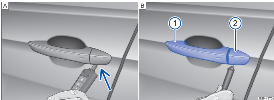
图 56 取下在驾驶员车门内车门锁的盖罩
