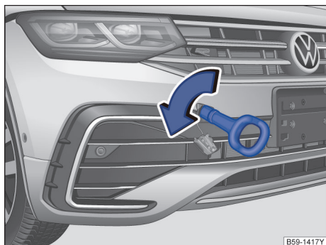
图 219 在保险杠的右前部：安装牵引环
